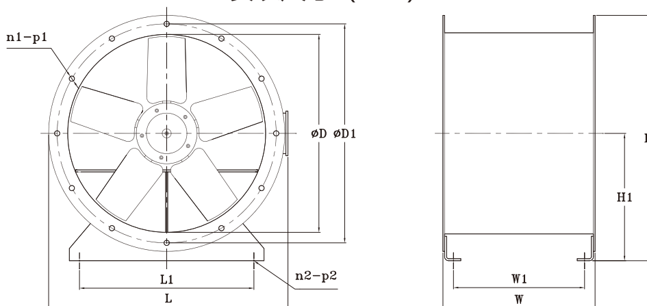
安裝尺寸 (mm)
