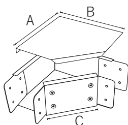
Front opening 正面蓋型
