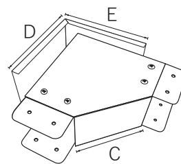
External opening 外開蓋型
