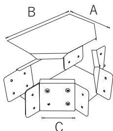
Front opening 正面蓋型
