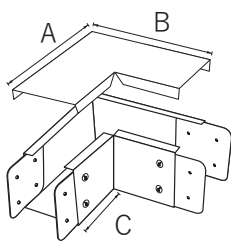
Front opening 正面蓋型
