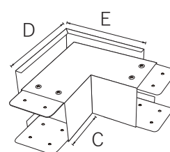
External opening 外開蓋型
